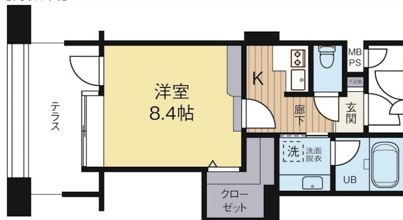
【間取り図】
