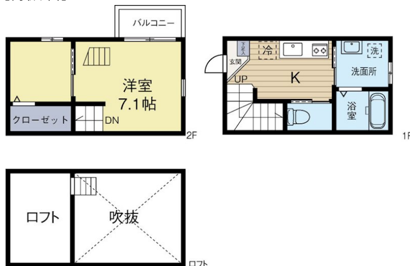
【間取り図】
