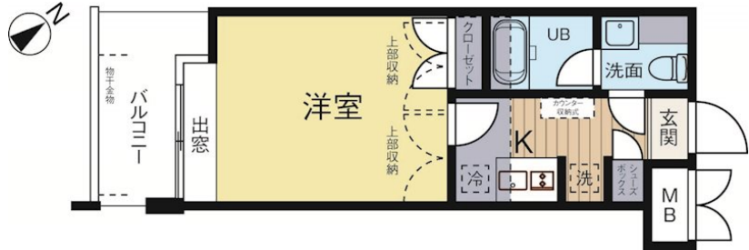
【間取り図】
