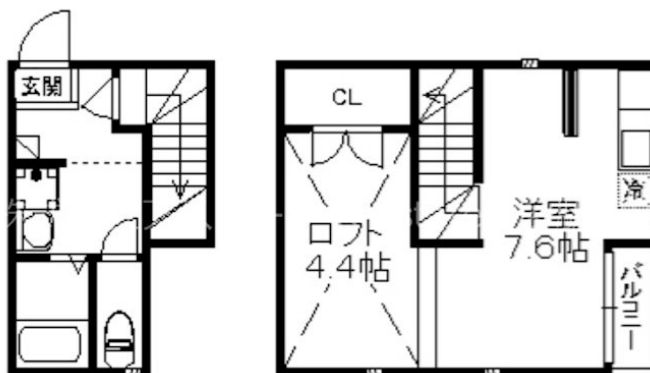
【間取り図】
