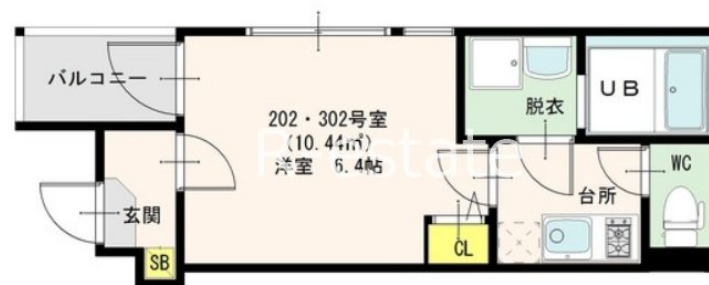
【間取り図】
