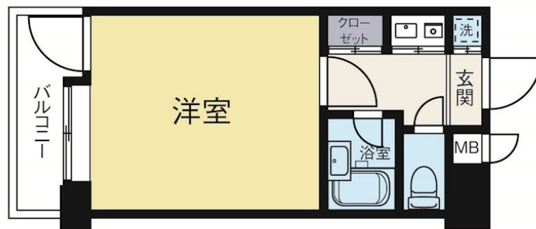
【間取り図】
