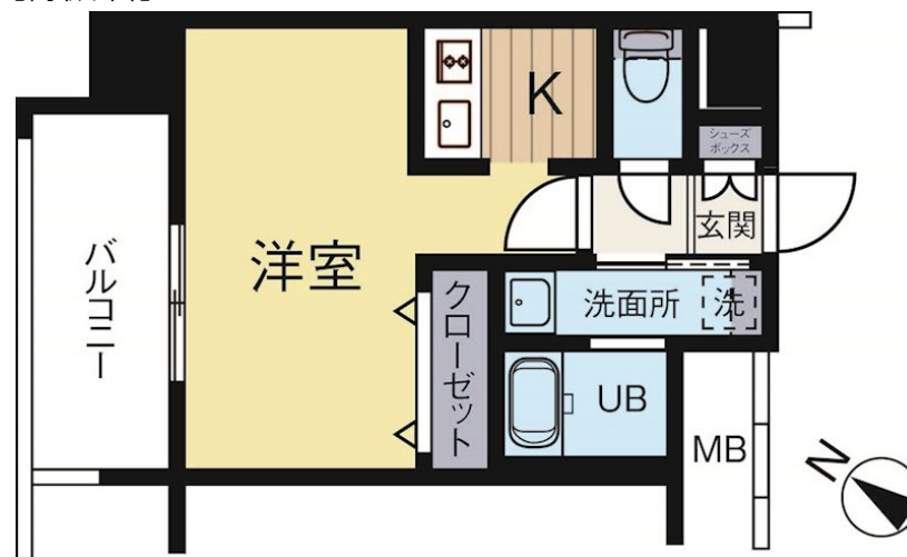
【間取り図】
